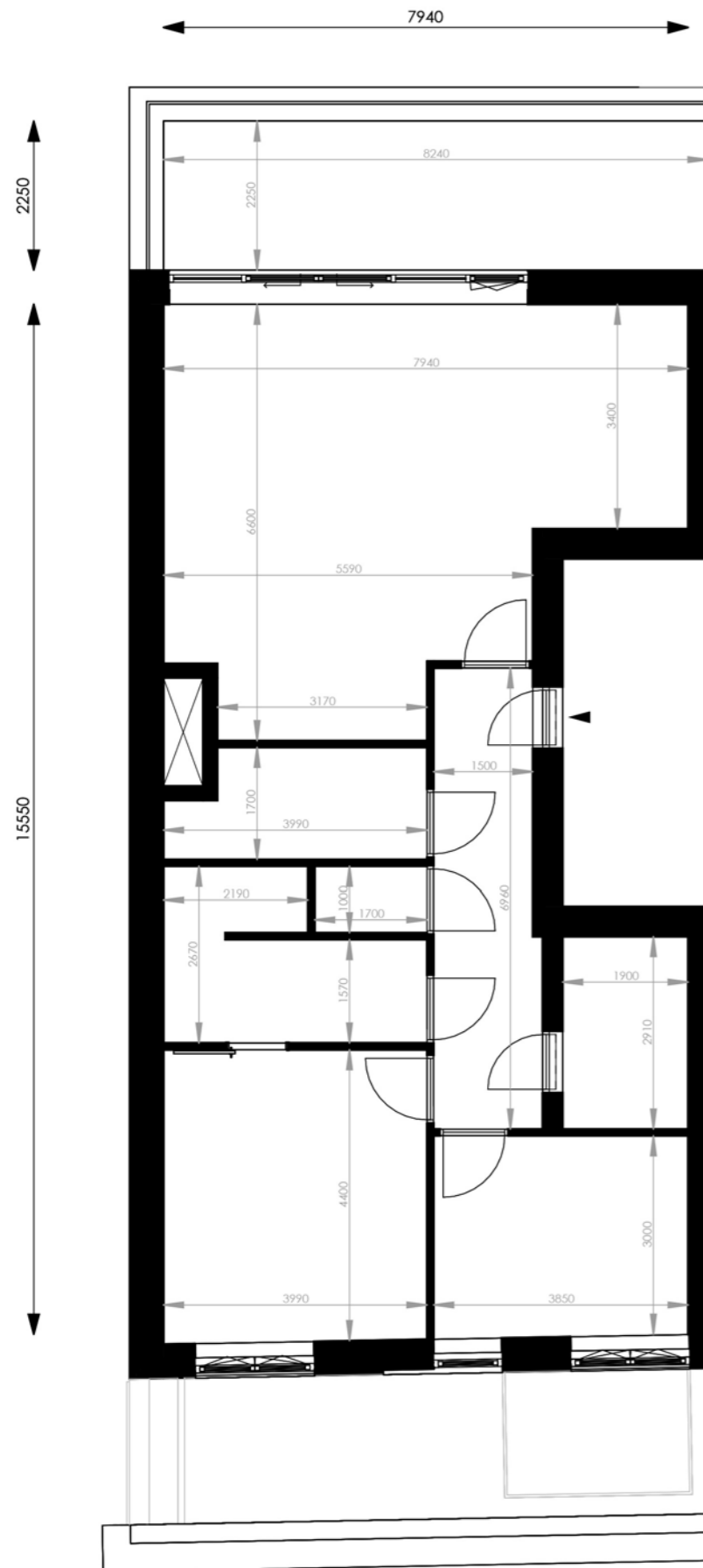
Appartement 3.11 | 1:100
